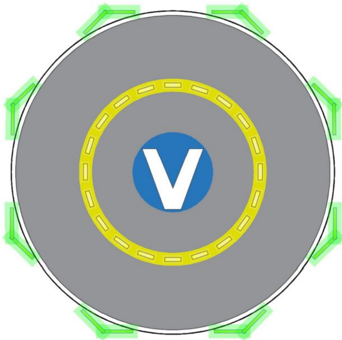
Слика Е-34. Нивои сегмената светала од тачкастих извора (ASPSL), односно светлосни панели (LPs) вертидрома у нивоу са земљом (зона приземљења и узлета (TLOF) кружног облика)
