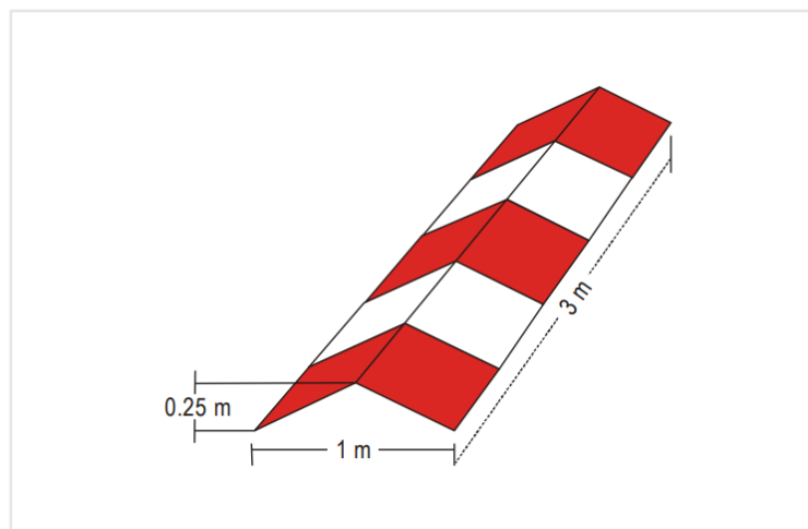
Слика Е-7. Маркер ивице зоне завршног прилаза и полетања типа полетно-слетне стазе ( runway-type FATO )
