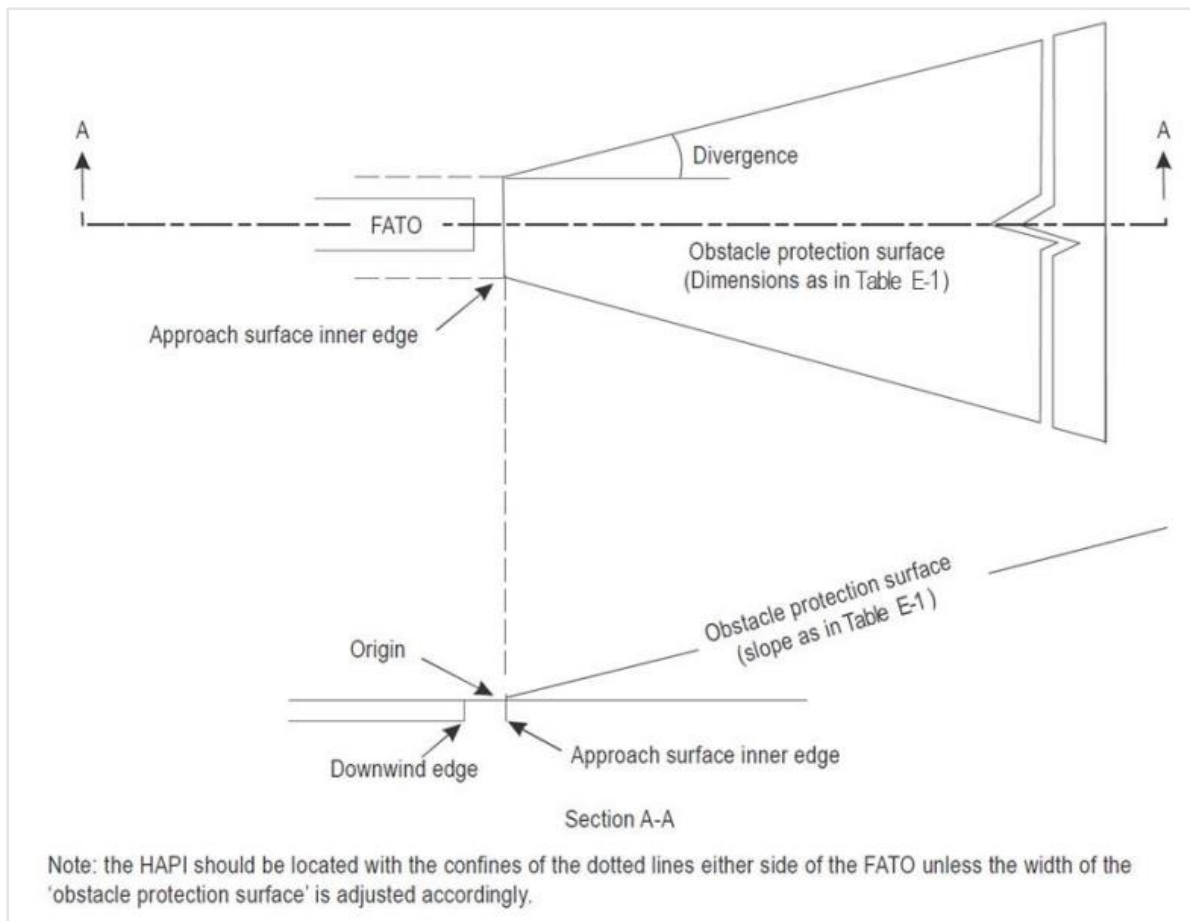
Слика Е-24. Површ за заштиту од препрека
