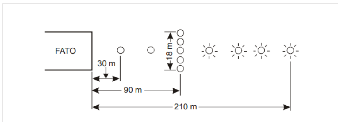
Слика Е-17. Систем прилазних светала
