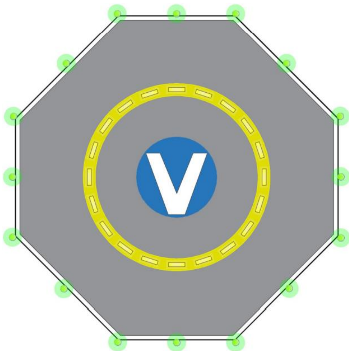
Слика Е-31. Светла вертидрома у нивоу са земљом и светла круга тачке додира/позиционирања (TDPC) (осмоугаона зона приземљења и узлета (TLOF))
