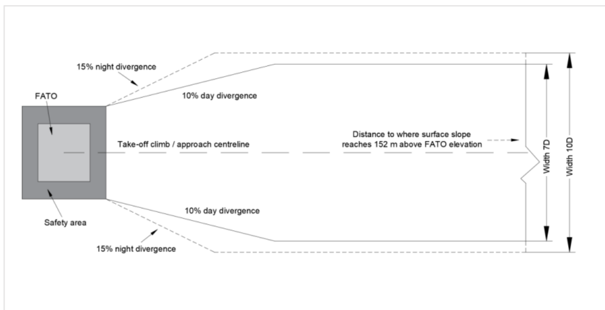
Слика Д-12. Ширине прилазно-одлетних површи (шематски приказ)
