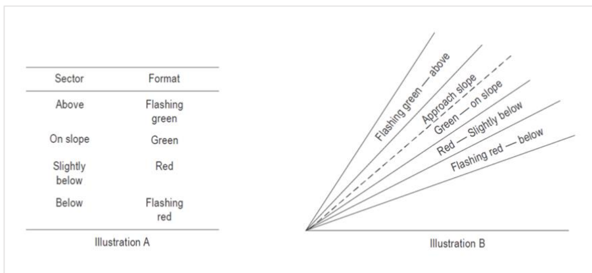
Слика Е-23. Формат сигнала визуелног показивача нагиба прилаза хеликоптера (HAPI)
