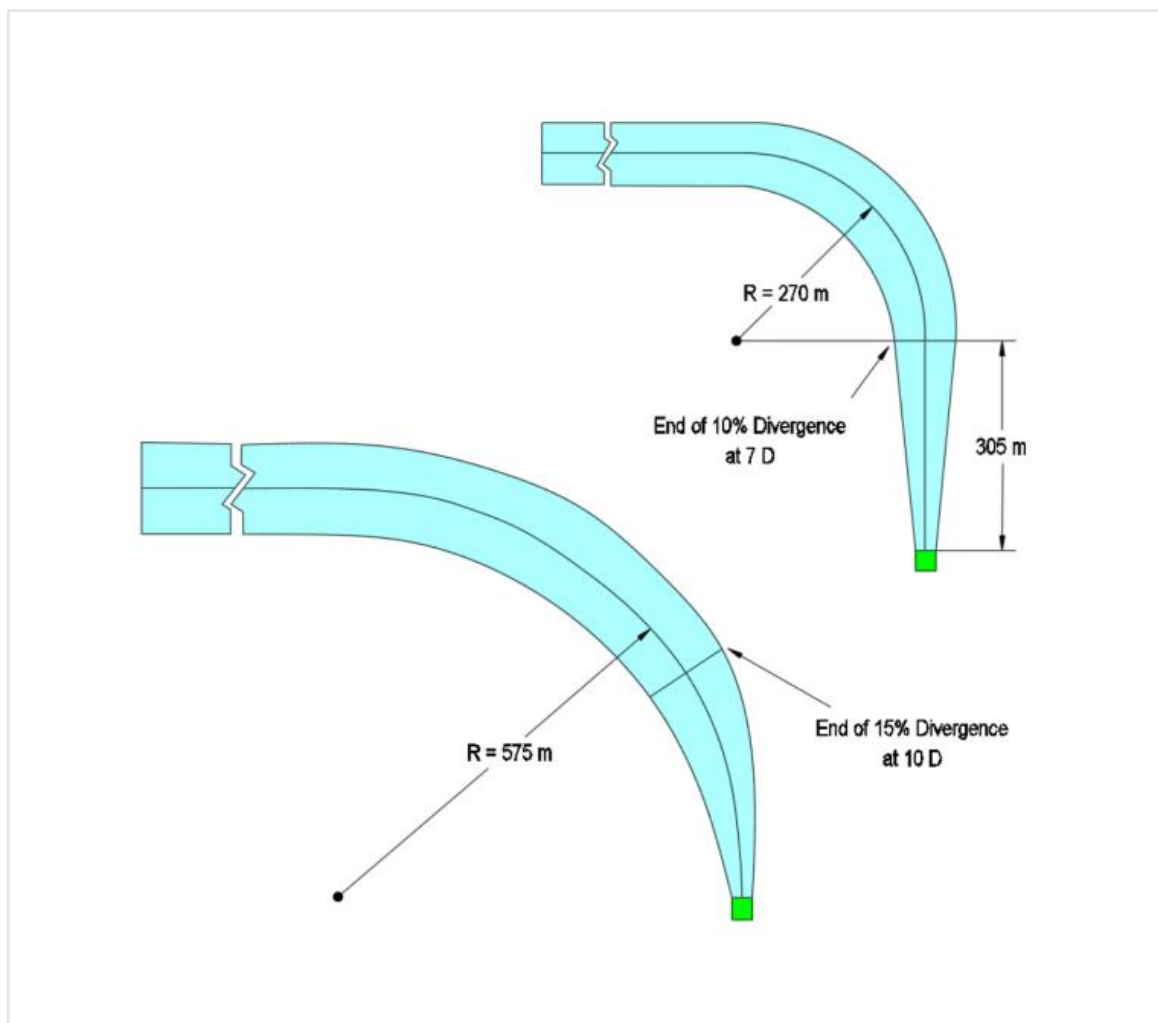
Слика Д-1. Прилазна и одлетна површ са закривљеном деоницом за све зоне завршног прилаза и полетања (FATOs)
