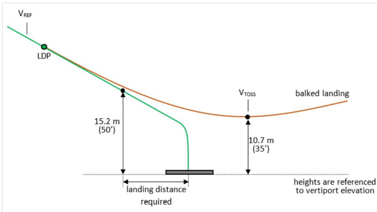
Слика Д-28. Путања за слетање
