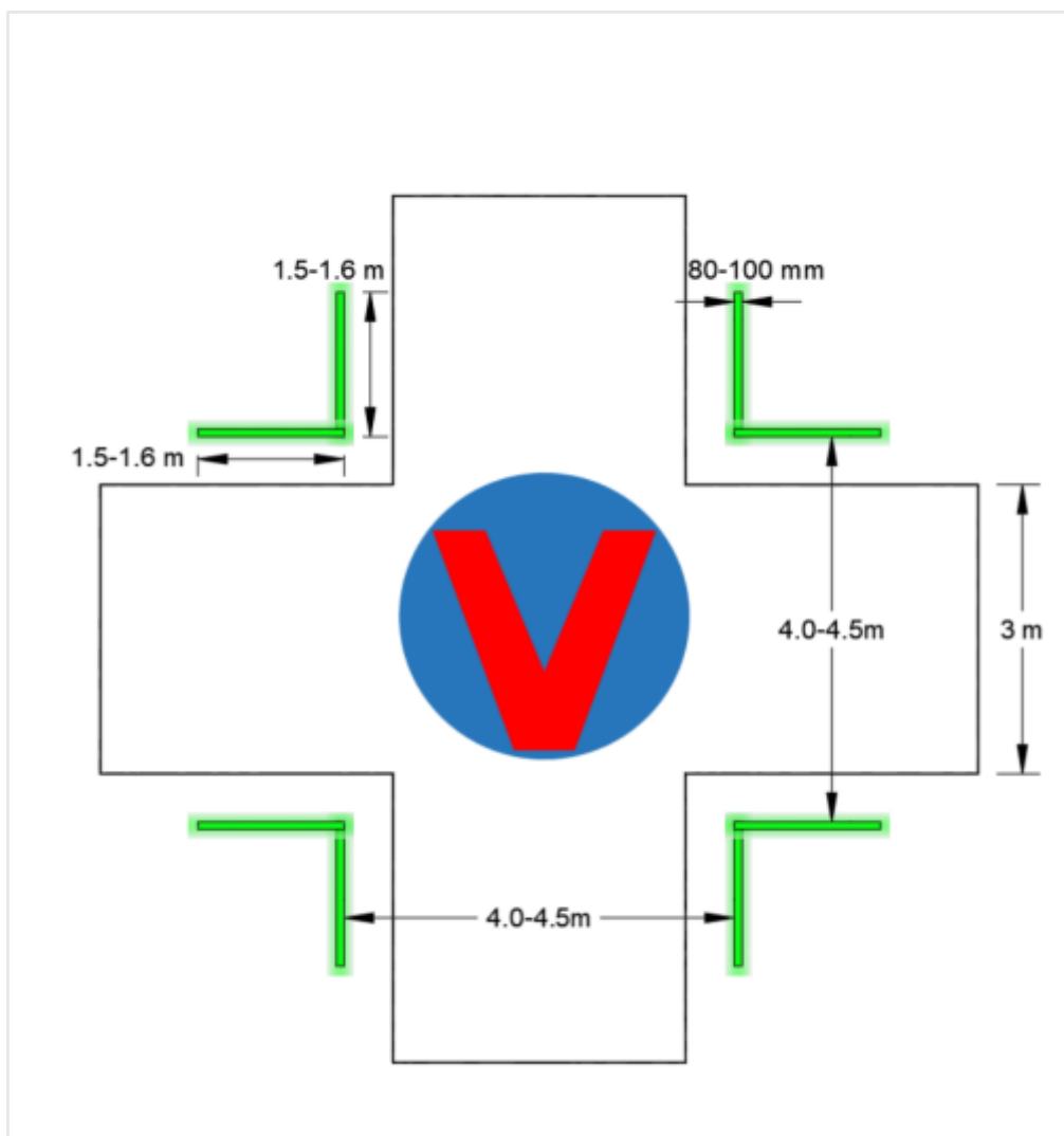
Слика Е-27. Светла крста на вертидрому
